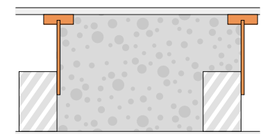
Unebenheiten der alten Balkenlage ausgleichen
