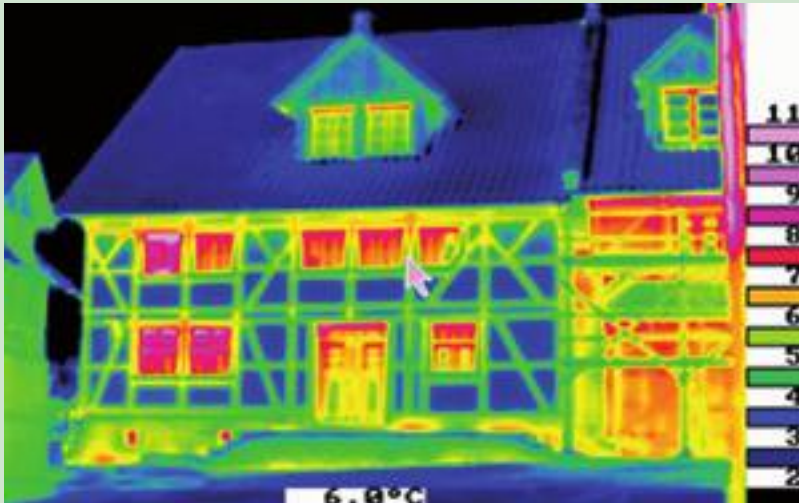
Thermografieaufnahme Objekt Quedlinburg
