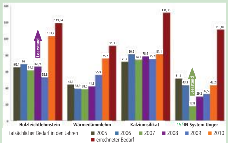
Quelle: Grafik 25 Entwicklung des Heizwärmebedarfs kWh/m² der Dämmvarianten von 2005 bis 2010 im Vergleich zu dem errechneten Jahresbedarf (Deutsches Fachwerkzentrum Quedlinburg)
